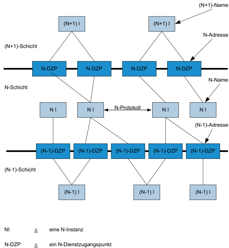
Abb. 1.2-2: Kennzeichnung der N-Instanzen durch N-Name und der N-Dienstzugangspunkte durch die N-Adresse
