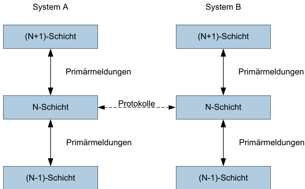
Abb. 1.2-1: Zu den Begriffen Schicht, Primärmeldungen und Protokolle
