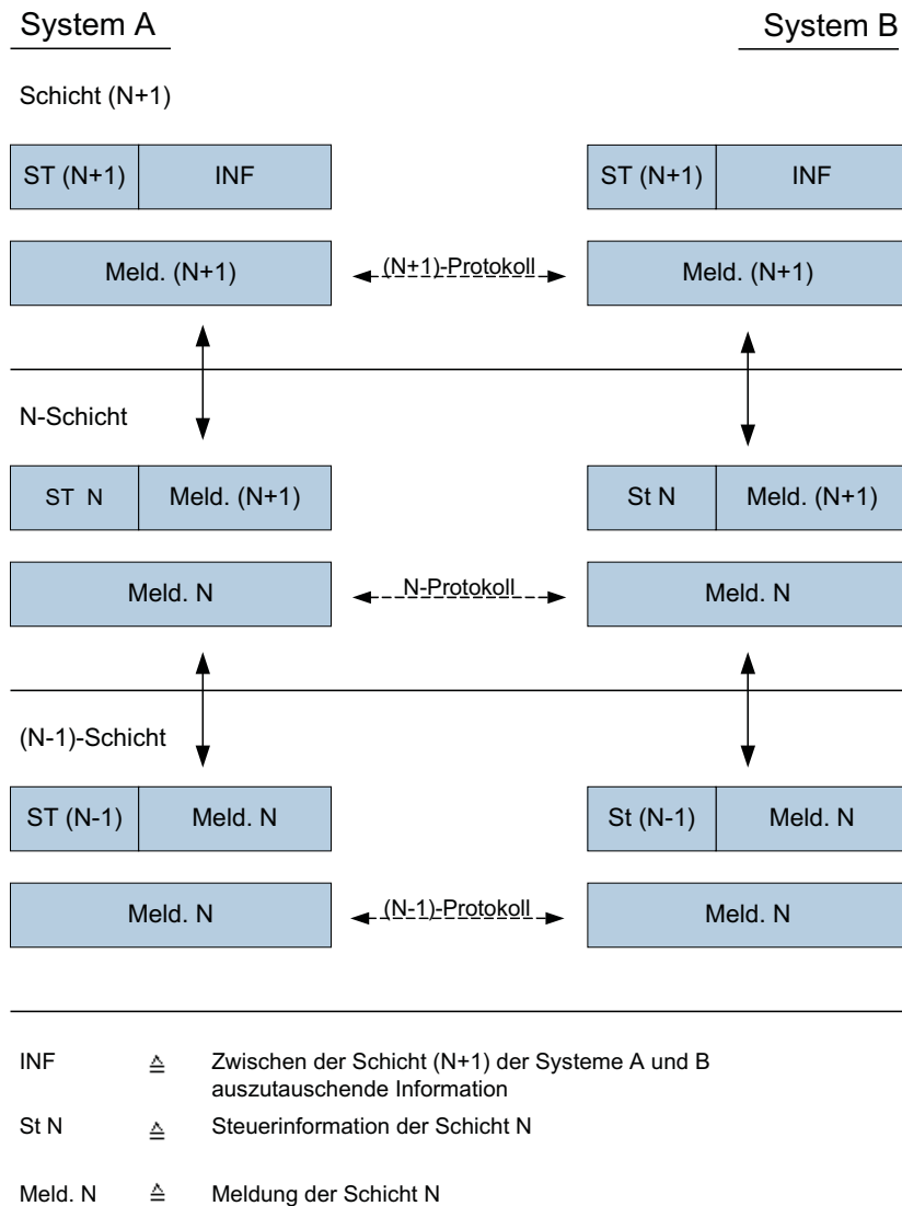
Abb. 1.2-7: Formate der Meldungen bei der Kommunikation zwischen Systemen
