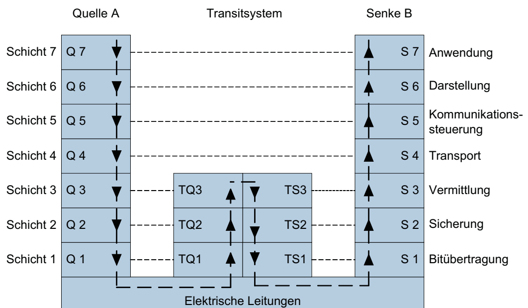
Abb. 1.1-2: Kommunikationsaufgaben bei der Briefübermittlung von A nach B nach dem OSI-Modell
