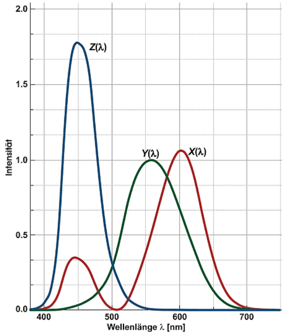
Abb. 1.3-4: Normenspektralwertkurven für den farbmetrischen Normalbeobachter ( 2^\circ )
