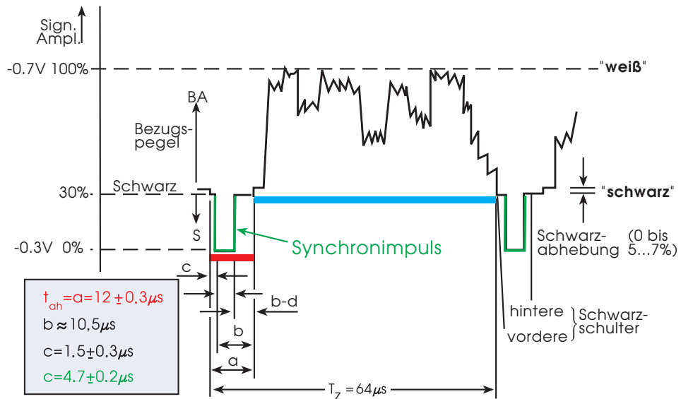
Abb. 1.4-4: FBAS-Signal
