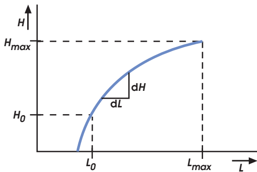
Abb. 1.2-3: Weber-Fechnerisches Gesetz
