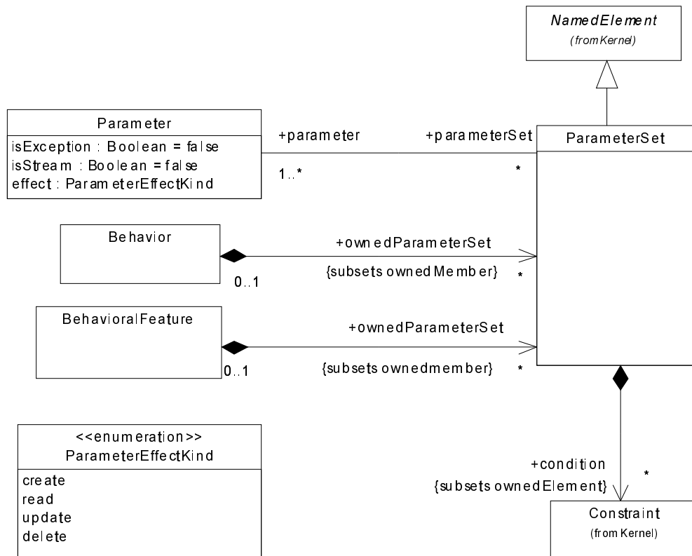
Figure 192 Parameter sets
