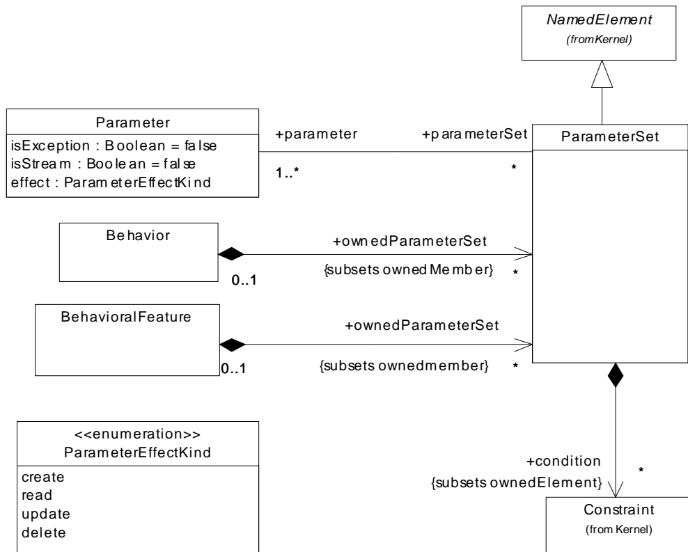
Figure 12.18 Parameter sets
